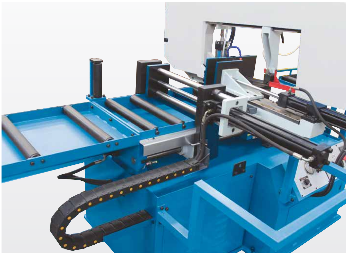
Мощные гидравлические тиски обеспечивают зажатие и подачу заготовок
